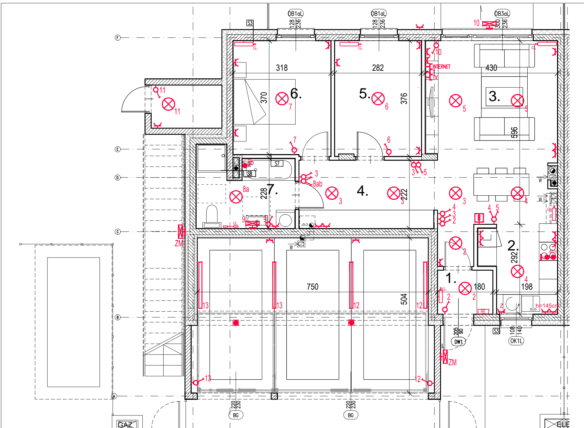
RZUT PARTERU
