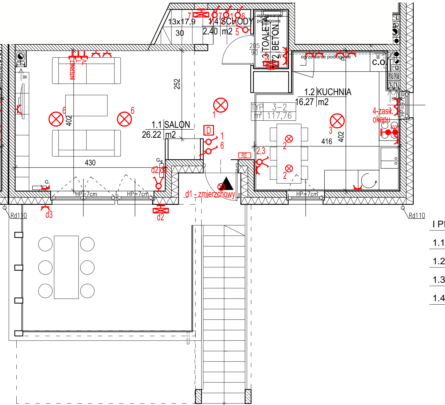
SKALA 1:66 I PIĘTRO
